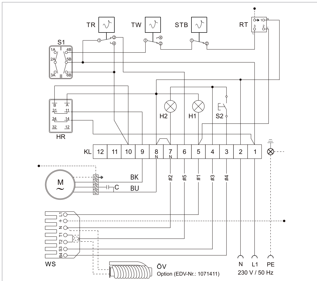
Abb. 3: Elektrisches Anschlussschema
